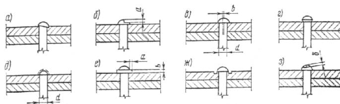
Рис. 8.1 Дефекты заклепок в соединении:
