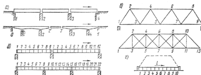
Рис. 1.1. Схема обозначения элементов искусственного сооружения: а - опор пролетных строений; б - диафрагм и панелей; в - элементов сквозных ферм; г - звеньев труб. Стрелкой показано направление хода километража для мостов
